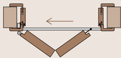
DVEŘE SKLÁDACÍ S POLODRÁŽKOU A VODICÍ LIŠTOU
