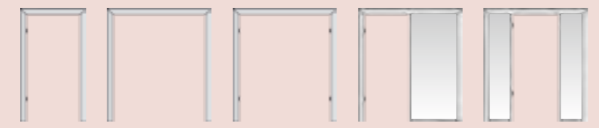
Zarge DIN links Durchgangszarge Doppeltürzarge Zarge DIN links mit Seitenteil rechts Zarge DIN links mit 2 Seitenteilen
